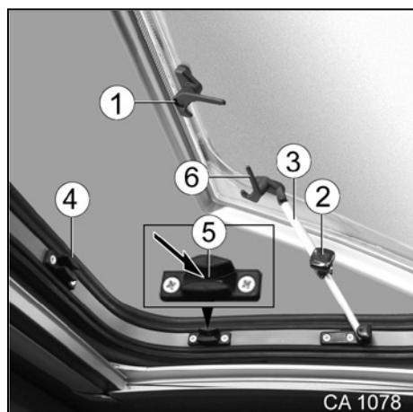
Afb. 64 Skyroof-dakluik
