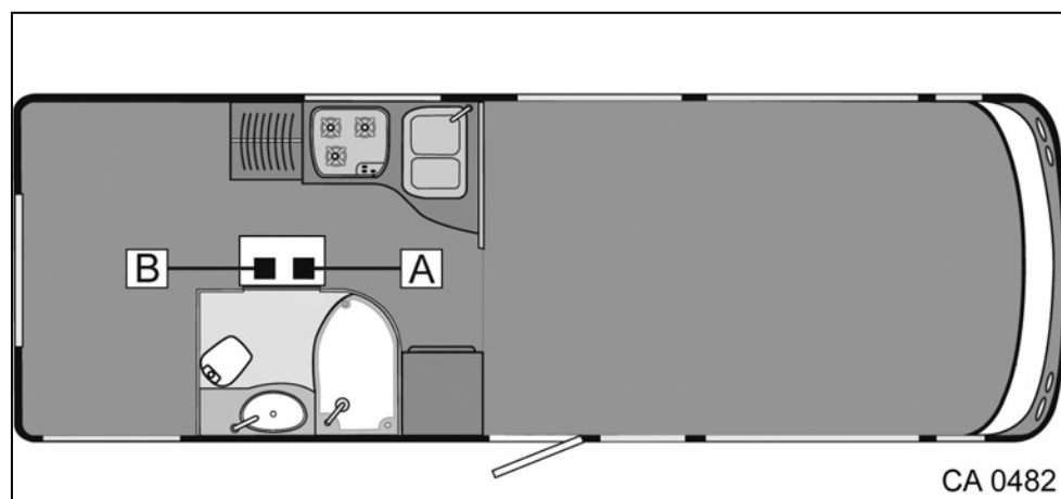
Afb. 171 Inbouwpositie waterstandsensoren
