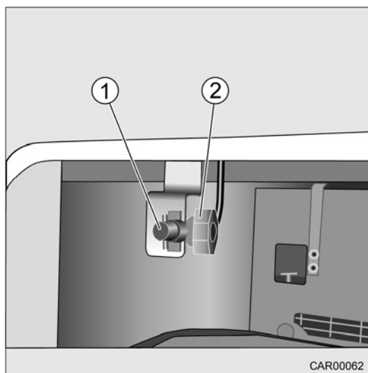
Afb. 117 Externe gasaansluiting
