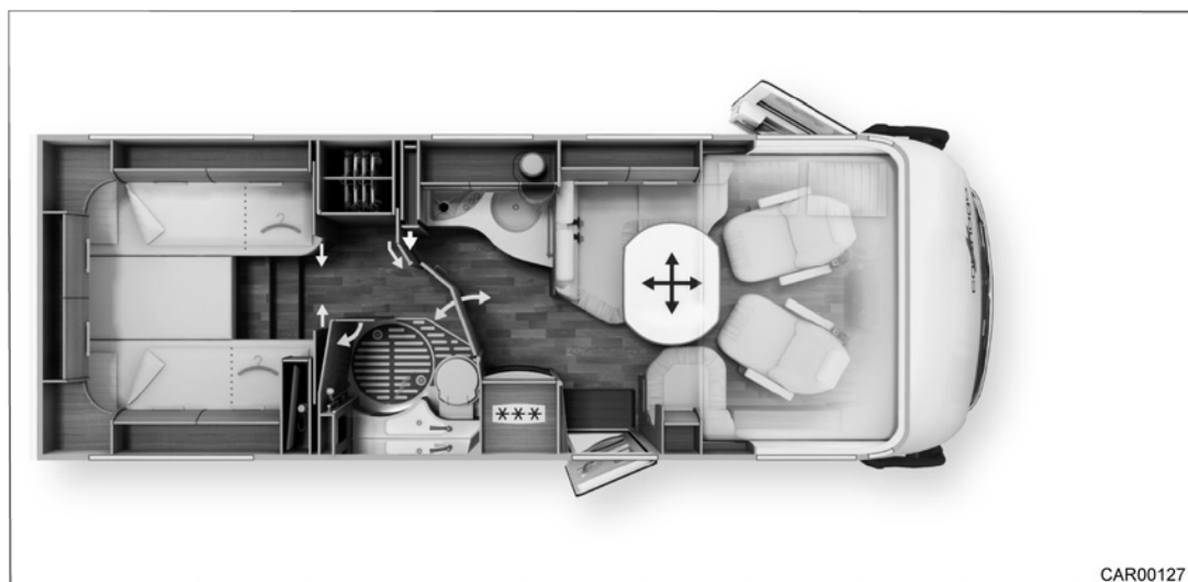
Afb. 87 Opbouw kleedruimte douche-badcombinatie en eenpersoonsbed in lengterichting
