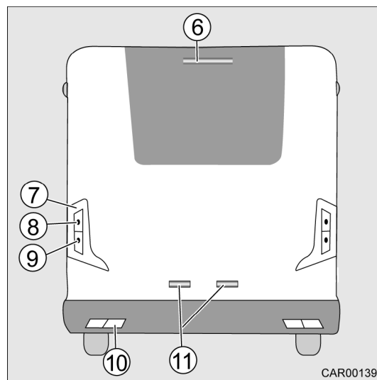
Afb. 181 Achterverlichting
