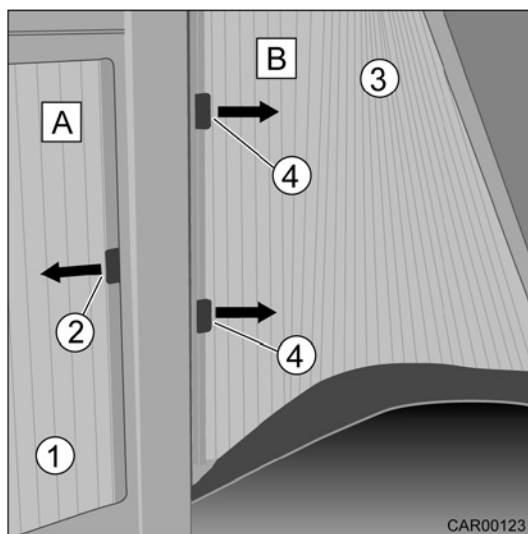
Afb. 82 Verduisteringsrolgordijn zij- raam/deur van de bestuurders- cabine
