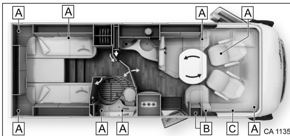
Afb. 163 Inbouwpositie bij uitvoering met eenpersoonsbed
