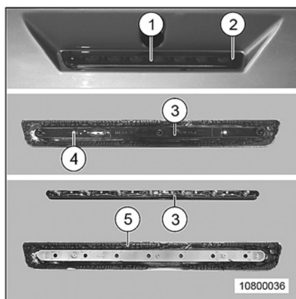
Afb. 191 Derde remlicht
