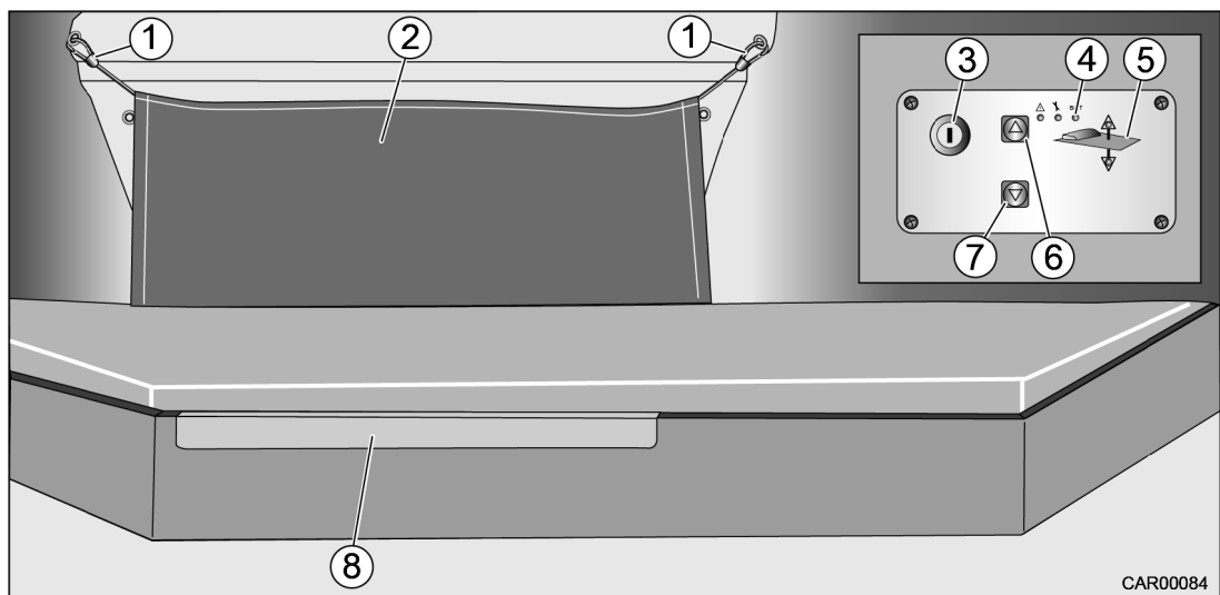
Afb. 76 Centraal opklapbed, elektrisch, verzonken
