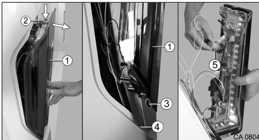
Afb. 187 Gloeilamp van de achterlichten vervangen
