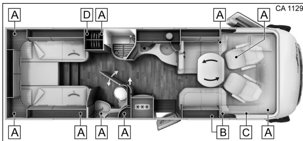
Afb. 164 Inbouwpositie uitvoering met eenpersoonsbed XL
