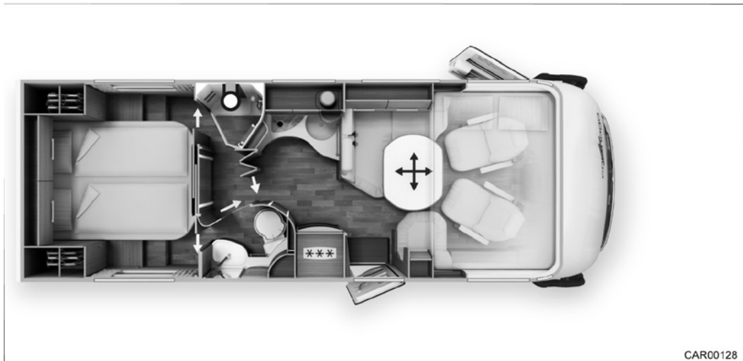
Afb. 91 Opbouw kleedruimte (ruimteverdeling) en queensbed
