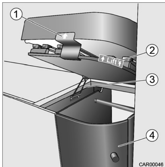
Afb. 78 Achterbed
