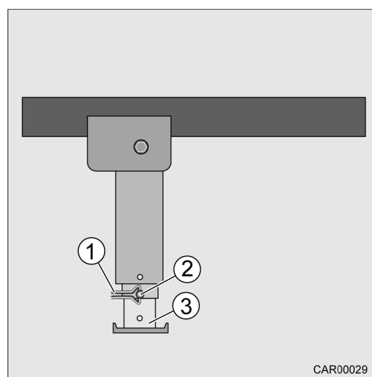
Afb. 38 Uitdraaibare hoeksteun achter Alko-chassis
