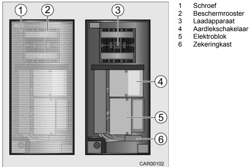
Afb. 111 Elektroblok in berging achterin
