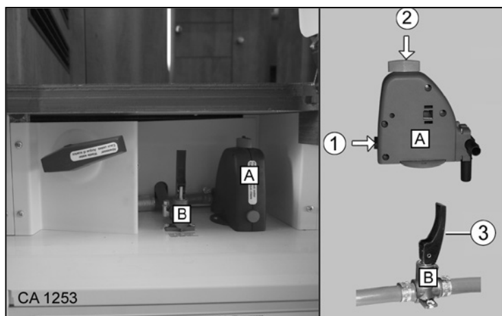
Afb. 146 Aftapkraan (A) boiler/aftapkraan (B) watersysteem
