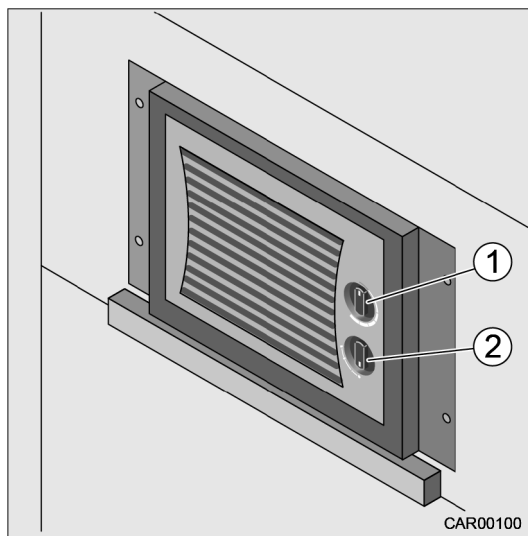
Afb. 122 Sirocco warmtewisselaar
