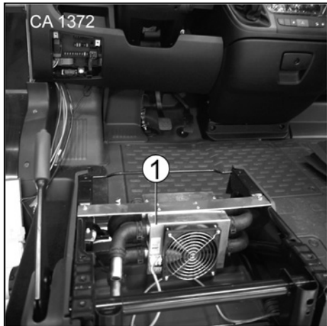
Afb. 127 Warmtebooster
