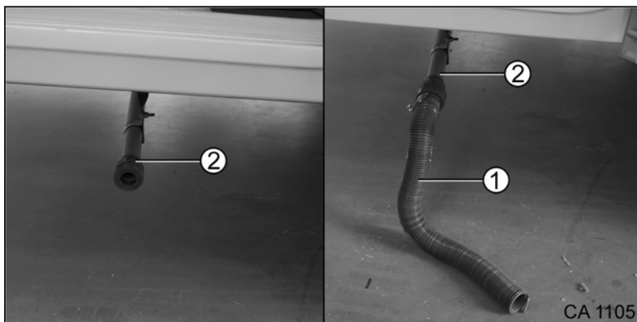
Afb. 151 Afvalwaterslangenset
