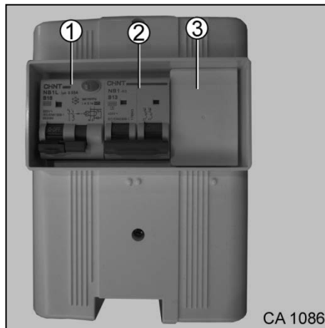
Afb. 106 Aardlekschakelaar
