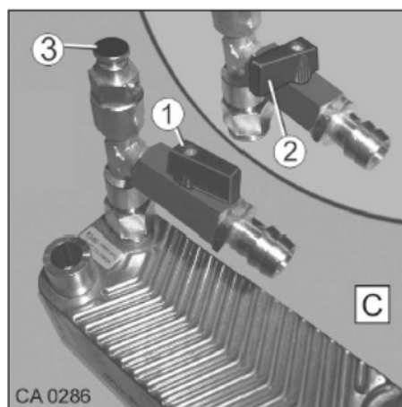
Afb. 170 Warmtewisselaar van de motor
