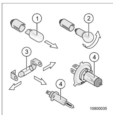
Afb. 183 Overzicht gloeilamptypen
