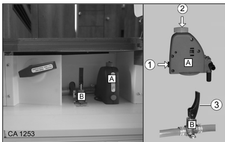
Afb. 147 Aftapkraan (A) boiler/aftapkraan (B) watersysteem
