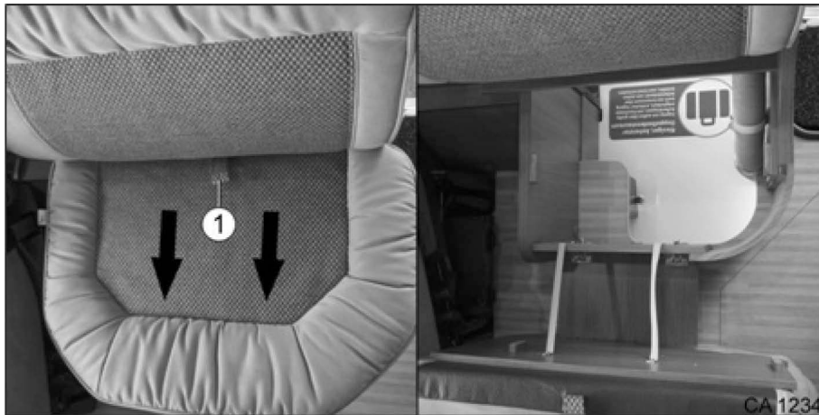
Afb. 71 Klapmechanisme korte zijzitbank
