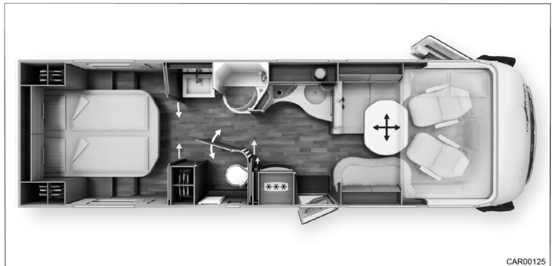
Afb. 92 Opbouw kleedruimte XL-badkamer
