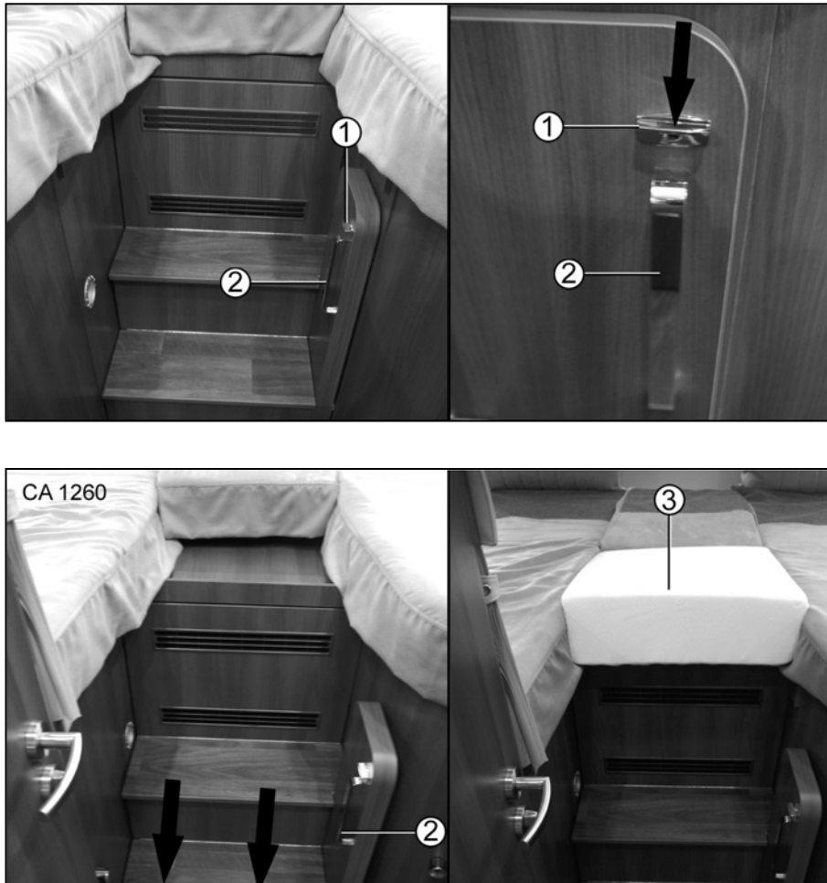
Afb. 79 Bedombouw
