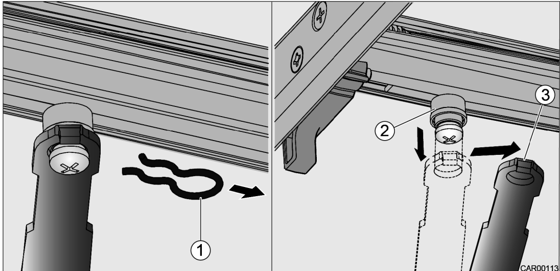
Afb. 12 Noodontgrendeling instaptrede
