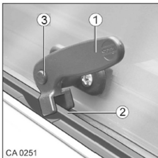
Afb. 57 Vergrendeling uitzetraam
