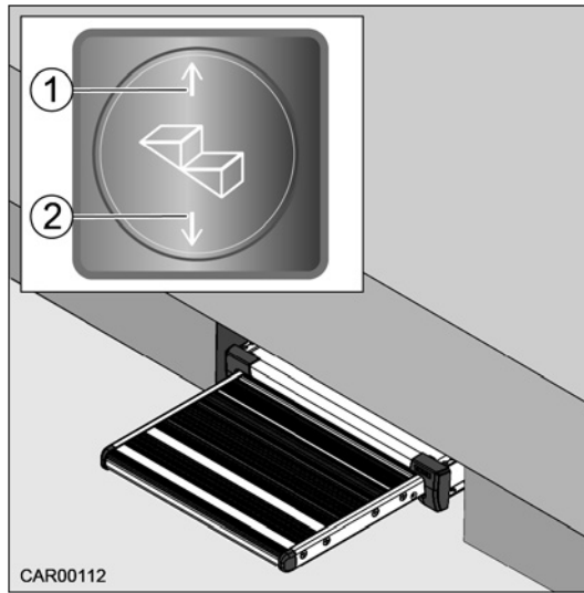
Afb. 9 Instaptrede slide-out
