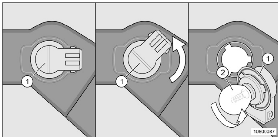
Afb. 186 Gloeilamp van de knipperlichten vervangen
