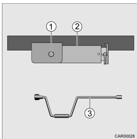
Afb. 37 Uitdraaibare hoeksteun achter Alko-chassis
