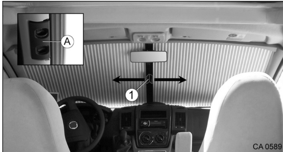
Afb. 84 Verduisteringsrolgordijn voorruit, geplooid
