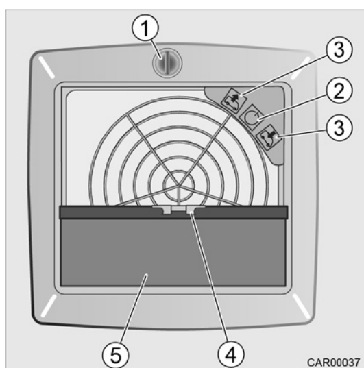
Afb. 66 Dakventilator elektrisch
