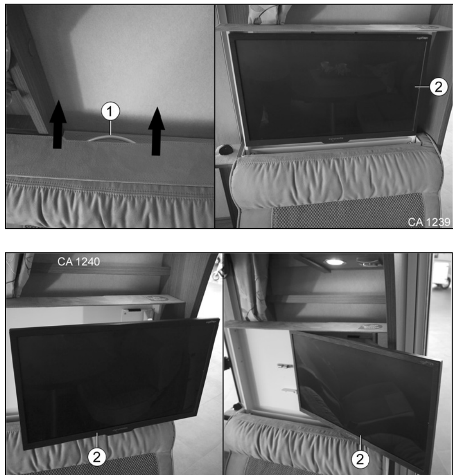
Afb. 137 TFT-uittreksysteem zijzitbank
