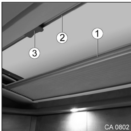
Afb. 65 Rolgordijnen Skyroof-dakluik
