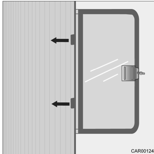
Afb. 83 Verduisteringsrolgordijn zijraam en passagierszijde
