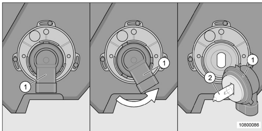
Afb. 184 Gloeilampen van dimlicht en grootlicht vervangen
