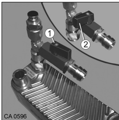
Afb. 125 Afsluitventiel warmtewisselaar
