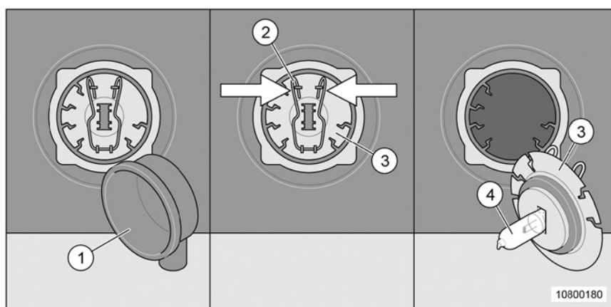
Afb. 185 Gloeilamp van de mistlamp vervangen
