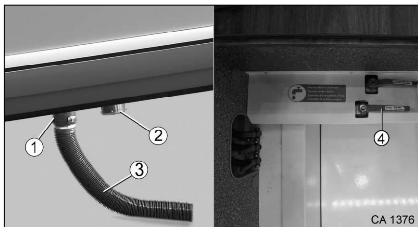
Afb. 159 Leging afvalwatertank
