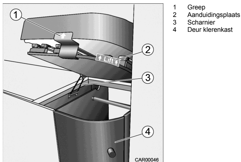
Afb. 91 Achterbed
