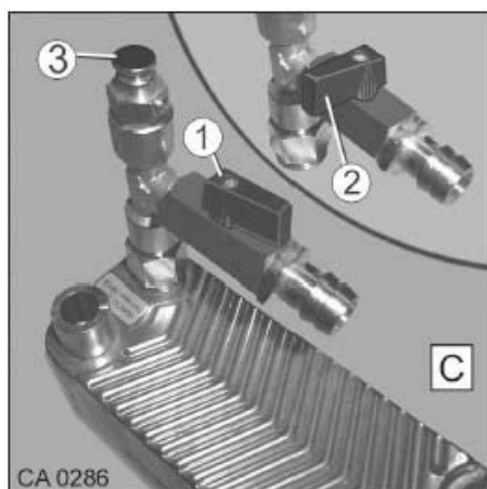
Afb. 181 Warmtewisselaar van de motor
