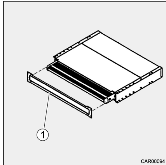
Afb. 23 Noodontgrendeling
