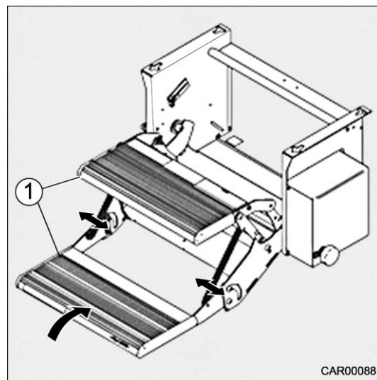
Afb. 16 Noodontgrendeling
