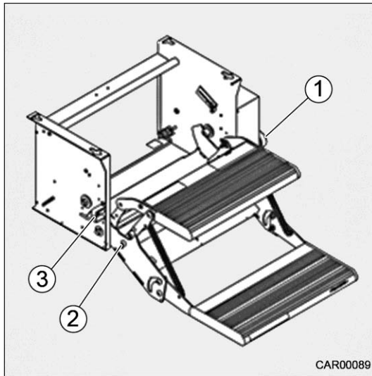
Afb. 17 Noodontgrendeling
