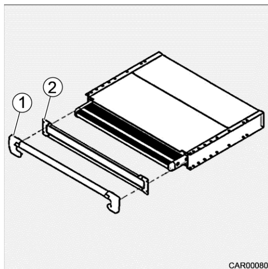
Afb. 9 Noodontgrendeling
