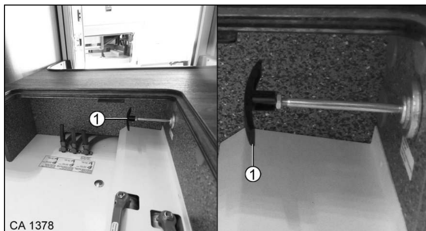
Afb. 164 Greep voor aftapschuif fecaliëntank
