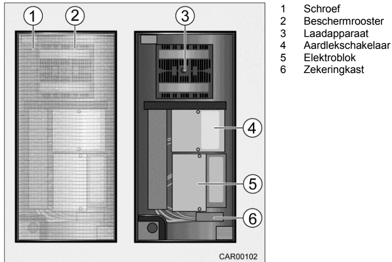
Afb. 120 Elektroblok in berging achterin
