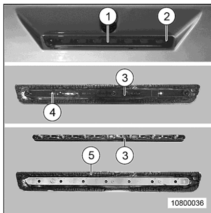
Afb. 204 Derde remlicht
