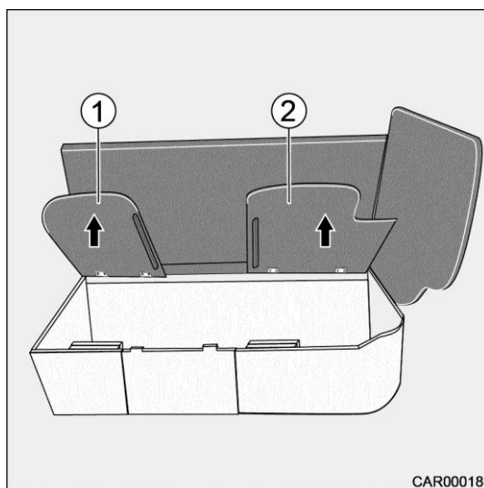
Afb. 43 Ombouw 5. Zitplaats
