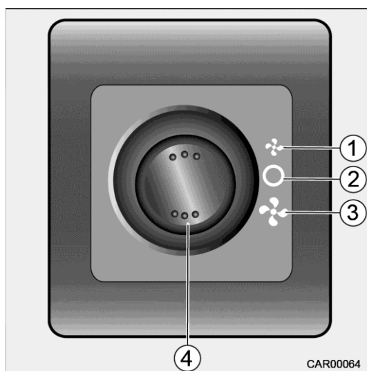
Afb. 137 Schakelaar voor warmtebooster
