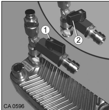
Afb. 133 Afsluitventiel warmtewisselaar
