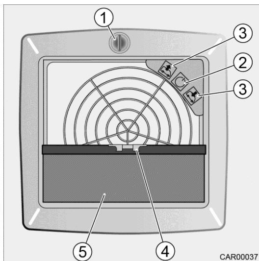
Afb. 77 Dakventilator elektrisch
