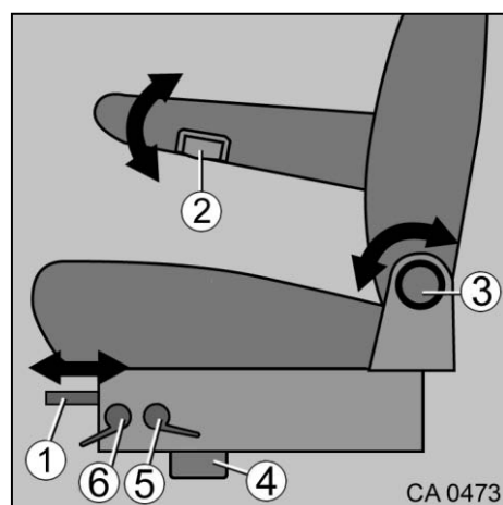
Afb. 33 Stoelverstelling met hoogte- en hellingshoekinstelling
