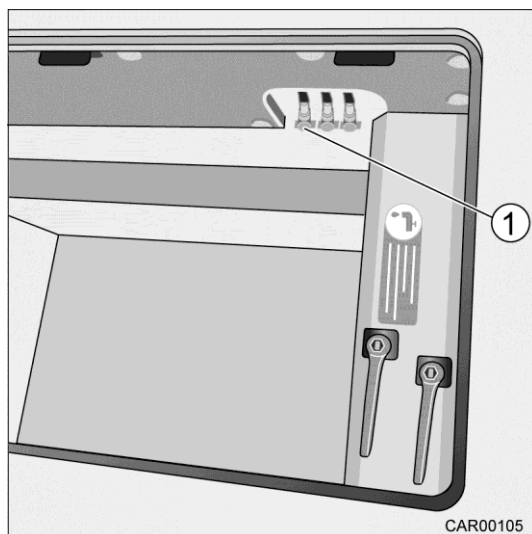
Afb. 155 Aftapkraan gewichtsreductie
