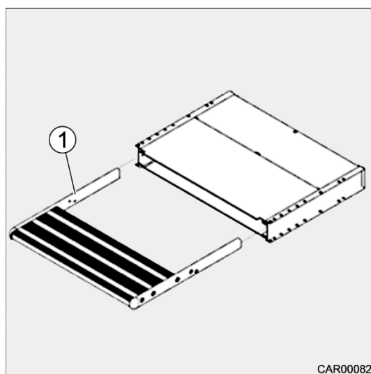
Afb. 11 Noodontgrendeling
