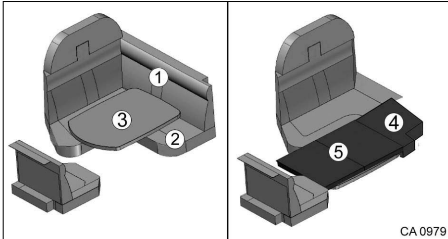
Afb. 83 Zitgroep tot bed ombouwen
