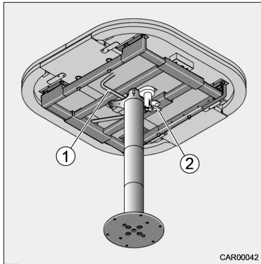
Afb. 80 Tafel neerlaatbaar
