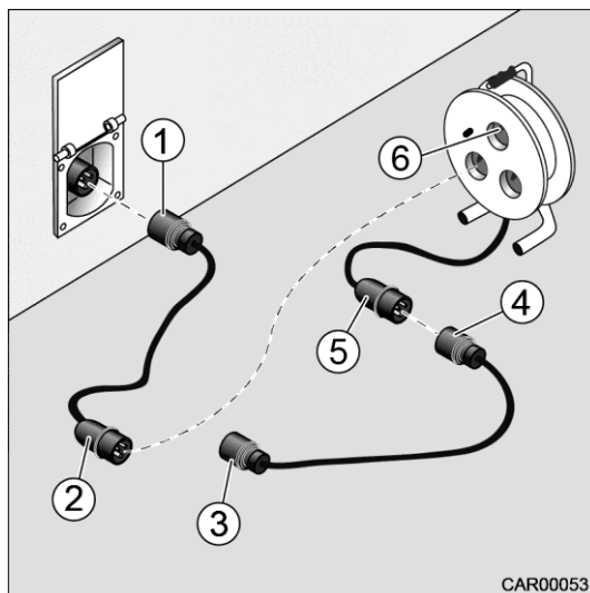
Afb. 116 Kabelaansluiting
