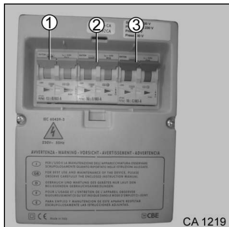
Afb. 115 Aardlekschakelaar
