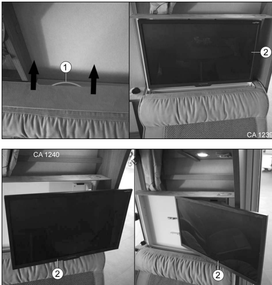
Afb. 147 TFT-uittreksysteem zijzitbank
