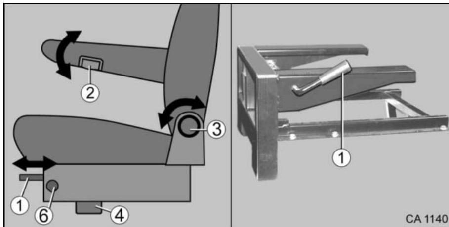
Afb. 34 Stoelverstelling met hoogte- en hellingshoekinstelling
