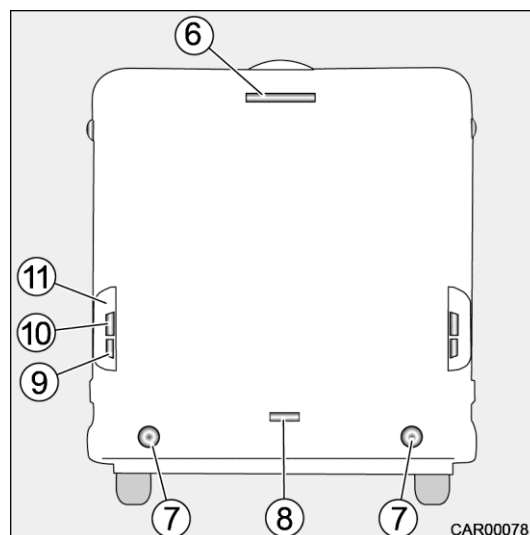
Afb. 194 Achterverlichting
