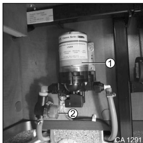
Afb. 172 Waterpomp
