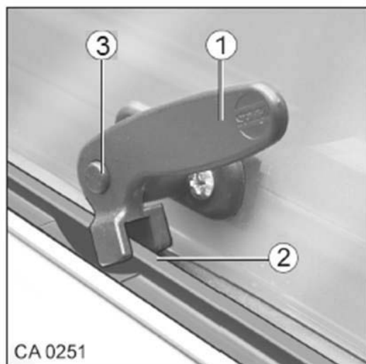
Afb. 70 Vergrendeling uitzetraam
