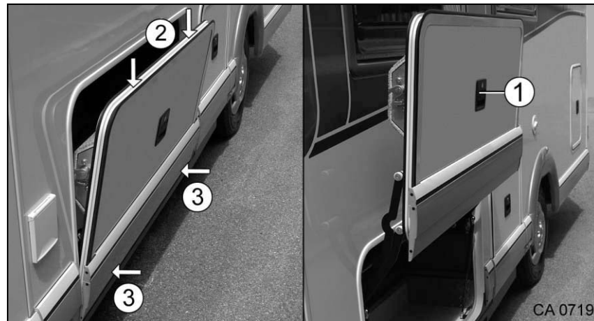
Afb. 66 Buitenkleppen openen/sluiten
