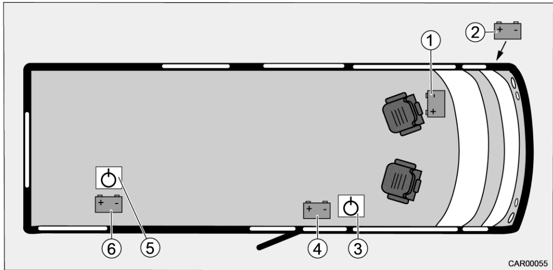
Afb. 117 Inbouwplaats accu's
