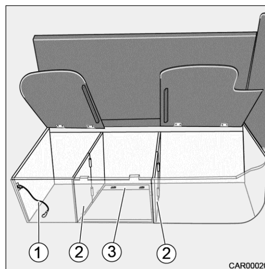
Afb. 44 Ombouw 5. Zitplaats
