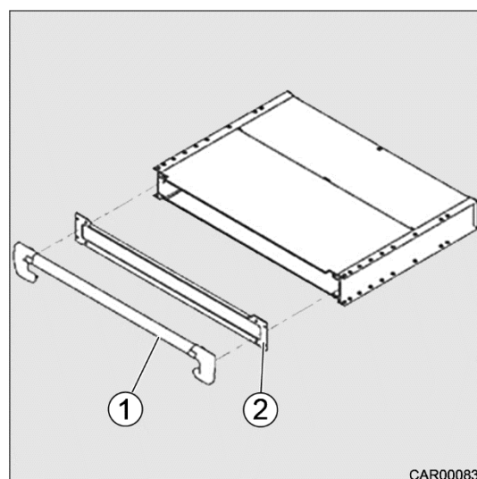
Afb. 12 Noodontgrendeling
