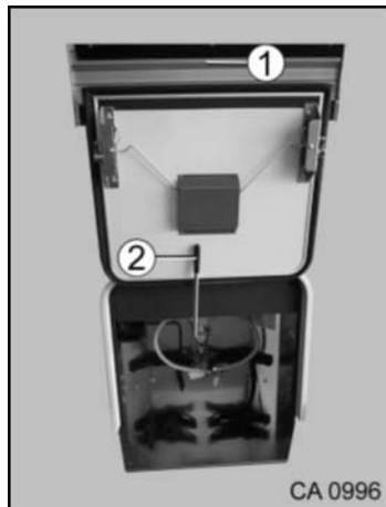
Afb. 65 Gaskastklep
