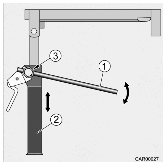
Afb. 55 Uitdraaibare hoeksteun achter s-plus
