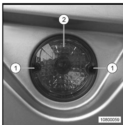
Afb. 202 Mistachterlicht
