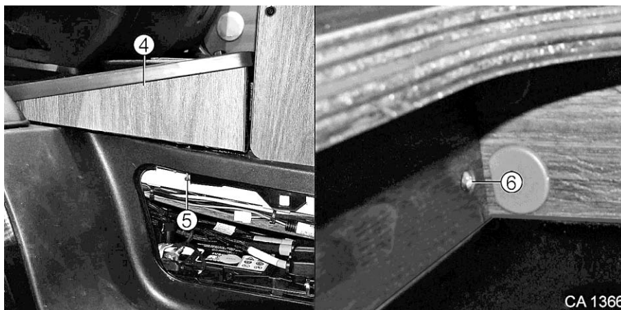
Afb. 206 Voertuigaccu vervangen
