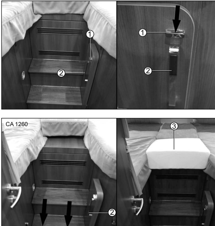
Afb. 92 Bedombouw
