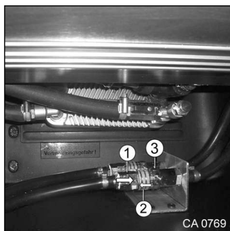
Afb. 135 Aansluitingen verwarmings- mat vloer bestuurderscabine
