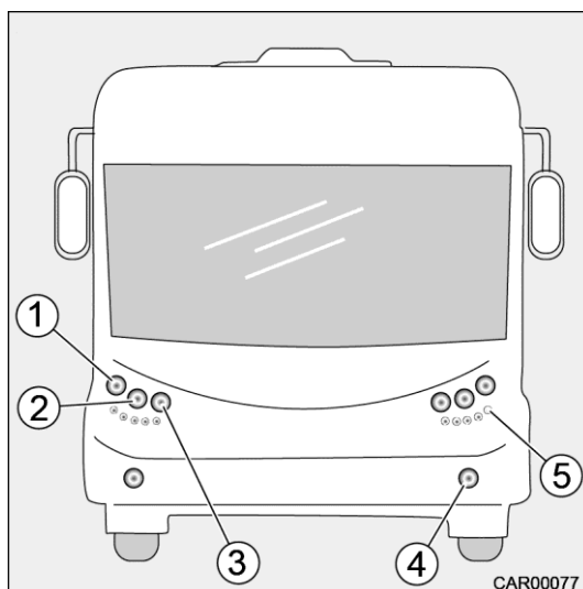
Afb. 193 Voorverlichting
