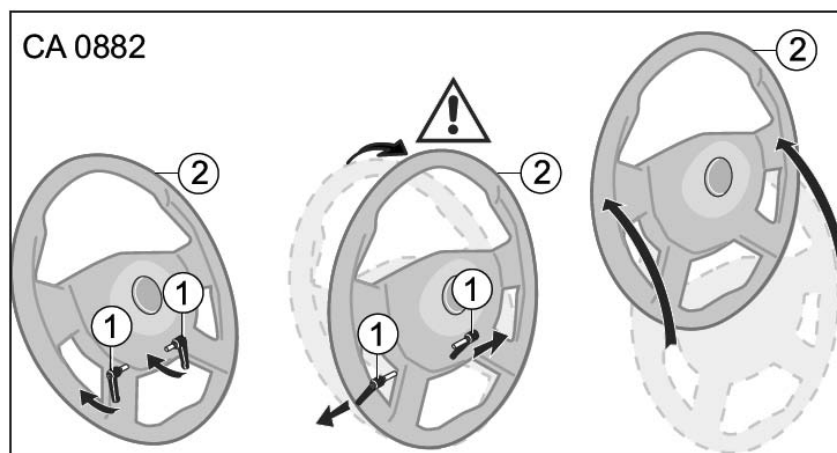
Afb. 87 Stuur wegdraaien
