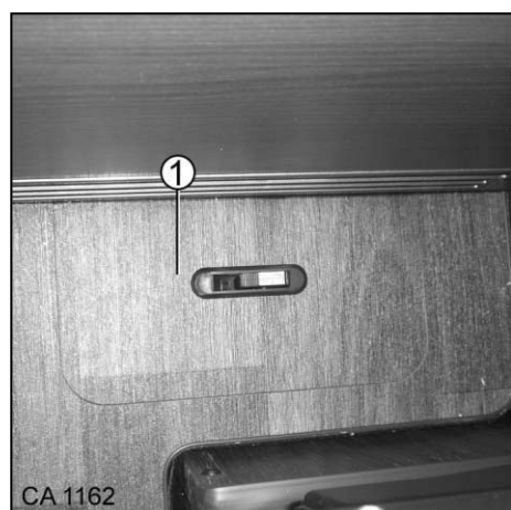
Afb. 132 Positie afsluitventiel warmtewisselaar Iveco
