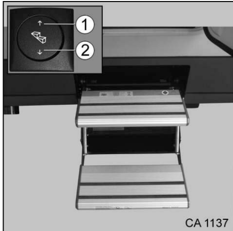
Afb. 13 Enkele instaptrede
