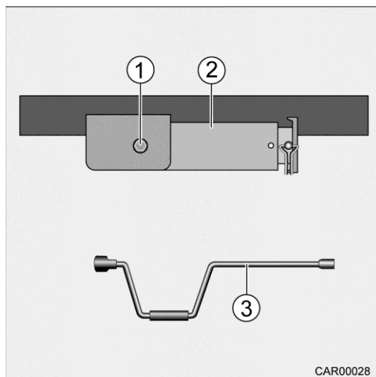
Afb. 56 Uitdraaibare hoeksteun achter e-line
