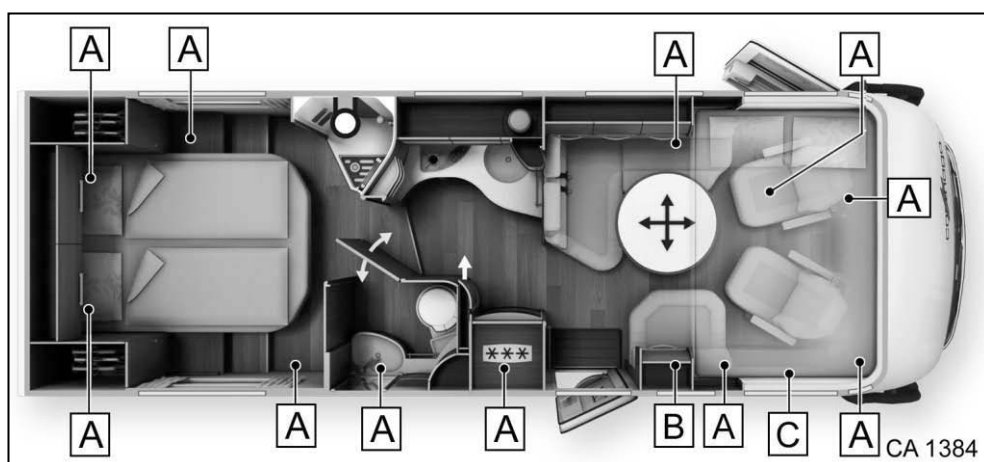
Afb. 177 Inbouwpositie queensize bed-uitvoering
