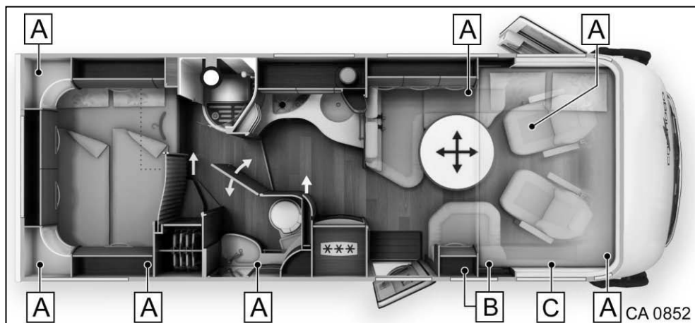
Afb. 176 Inbouwpositie tweepersoonsbed met ruime badkamer
