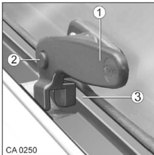
Afb. 69 Vergrendeling uitzetraam
