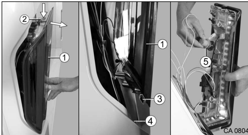
Afb. 200 Gloeilamp van de achterlichten vervangen
