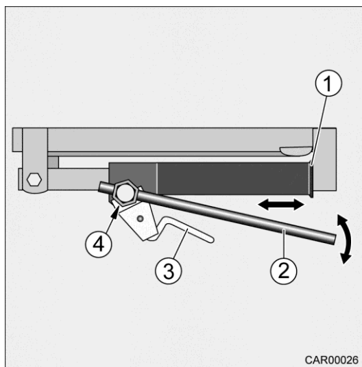
Afb. 54 Uitdraaibare hoeksteun achter s-plus
