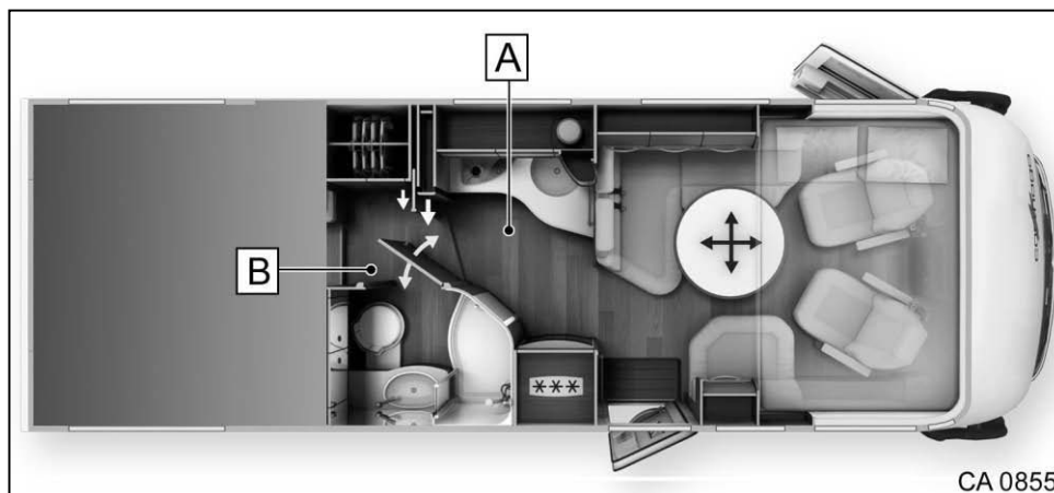
Afb. 182 Inbouwpositie waterstandsensoren
