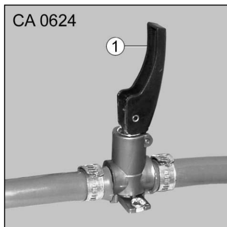
Afb. 138 Aftapkraan boiler
