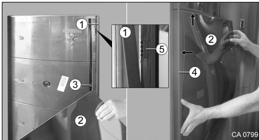
Afb. 141 Koelkastdeur ontgrendelen
