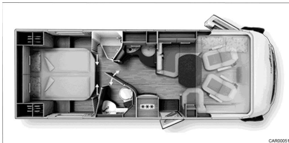
Afb. 98 Opbouw kleedkamer ruime badkamer (enkele deur)
