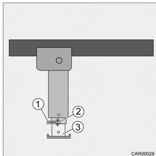
Afb. 57 Uitdraaibare hoeksteun achter e-line
