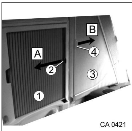
Afb. 95 Verduisteringsrolgordijn zijraam/deur van de bestuurderscabine
