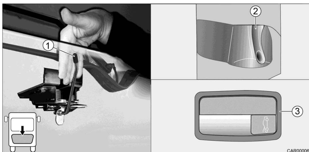
Afb. 24 Motorkap open maken
