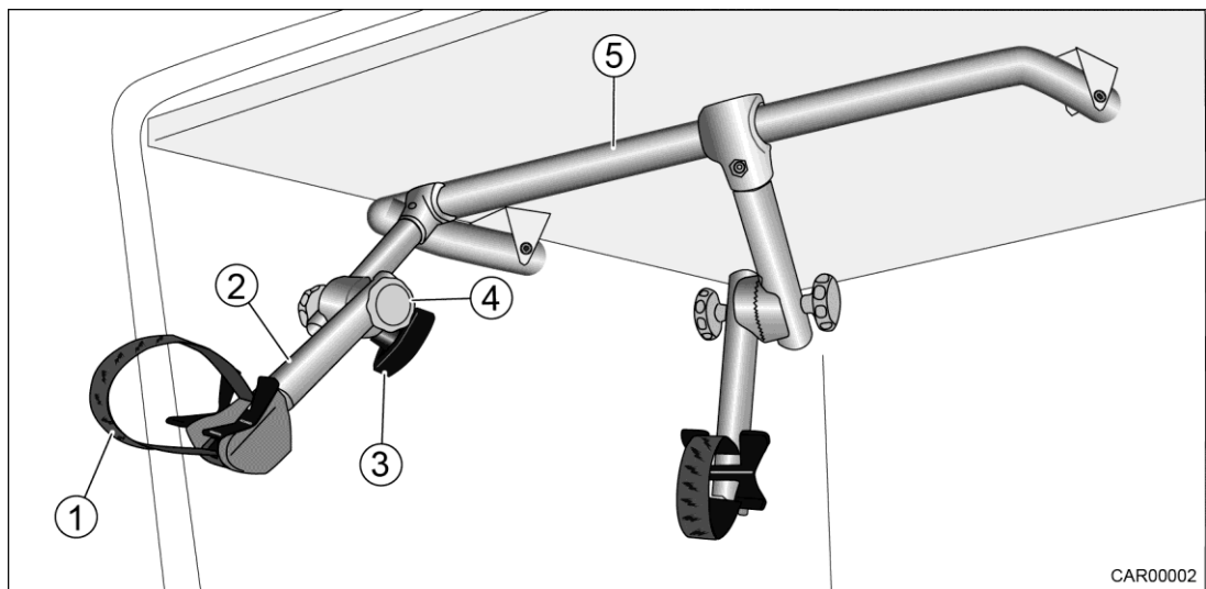
Afb. 4 Steunstangen berging voor elektrische fietsen
