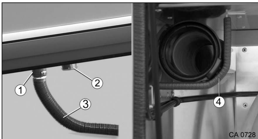
Afb. 158 Waterafvoer/opbergen van de aftapslang
