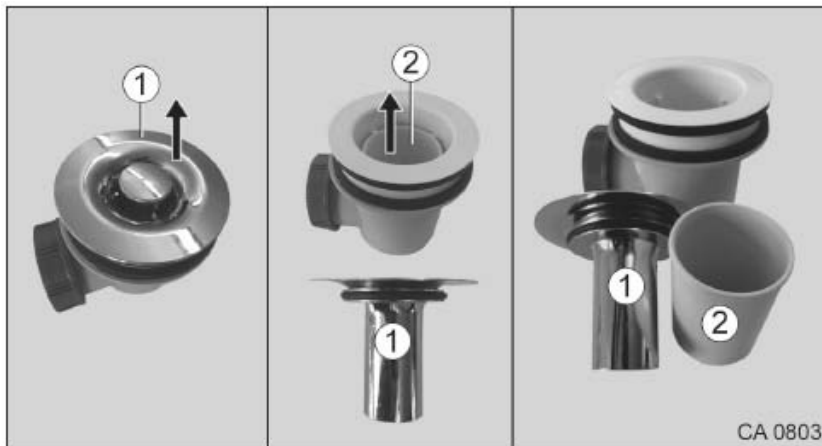
Afb. 161 Stankafsluiter, uitvoering met chromen afdekking
