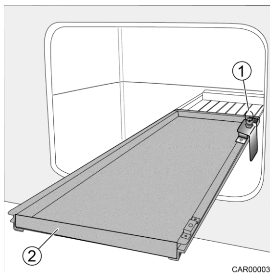
Afb. 2 Uitschuifstelsysteem
