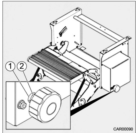
Afb. 18 Noodontgrendeling
