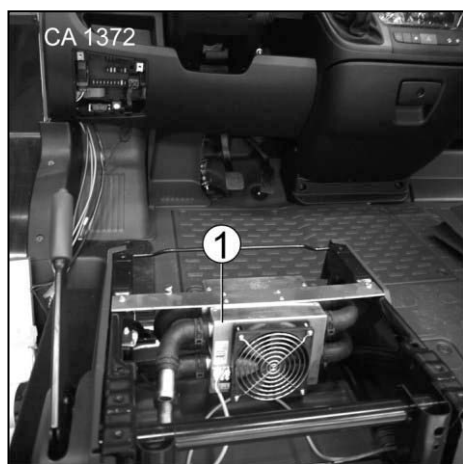
Afb. 136 Warmtebooster
