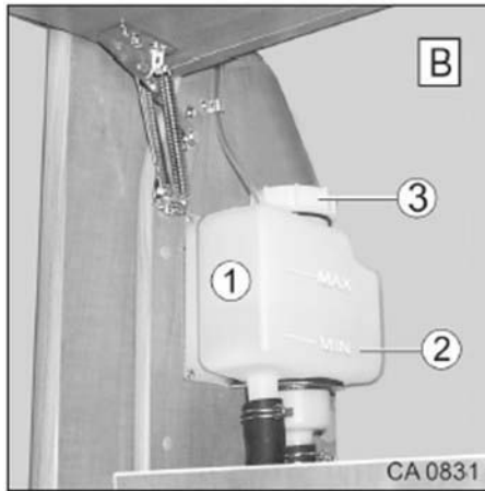
Afb. 180 Expansievat
