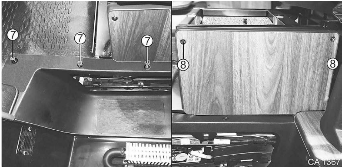
Afb. 207 Voertuigaccu vervangen
